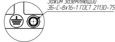
Н Заземление рамы агрегата
